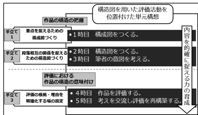
図1 単元構想図
